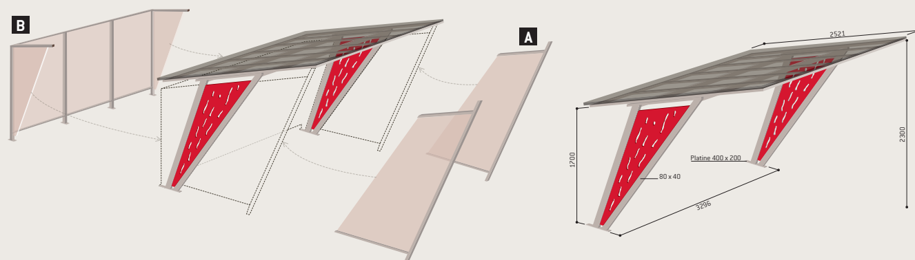
Modèle présenté : réf. 529630 gris Procity avec décor rouge 327 + appuis cycles réf. 297382
