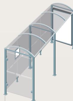
Lérins - Longueur 5000 Une vitrine 2000 + un bardage latéral 529339
