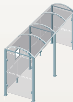
Noirmoutier - Longueur 5000 Deux bardages latéraux 529319
