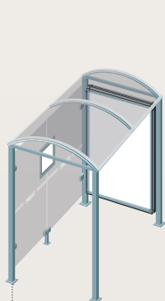
Ouessant - Longueur 2500 Une vitrine 2000 529328
